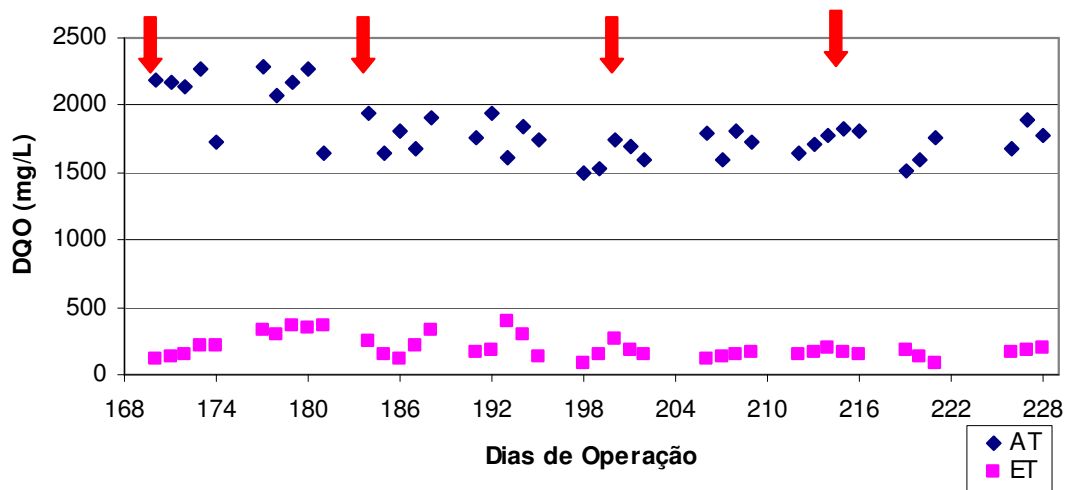
Figura 4.8: DQO T afluyente e efluente do biorreator Teste durante o período de choques quinzenais (indicados pelas setas em vermelho).
