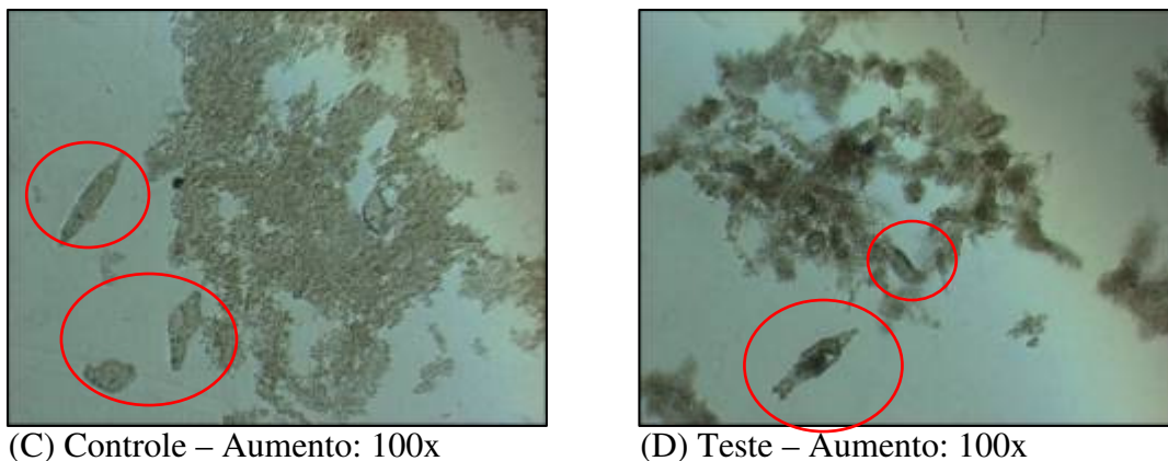
Figura 4.23: Fotos em campo claro dos flocos dos biorreatores Controle e Teste após o término dos choques semanais com 8 horas de duração.
