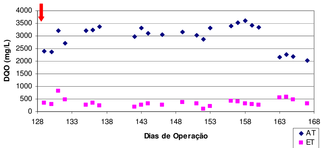
Figura 4.5: DQO T afluyente e efluyente do biorreator Teste após o primeiro choque (indicado pela seta em vermelho).
